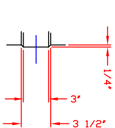
DETAIL 'A'--STIFFENER BAND SCALE: 1 1/2"=1'-0"
