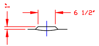
DETAIL 'B' (2) PL.
