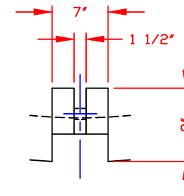
LIFTING LUG DETAIL (6) PLACES SCALE: 1"=1'-0"
