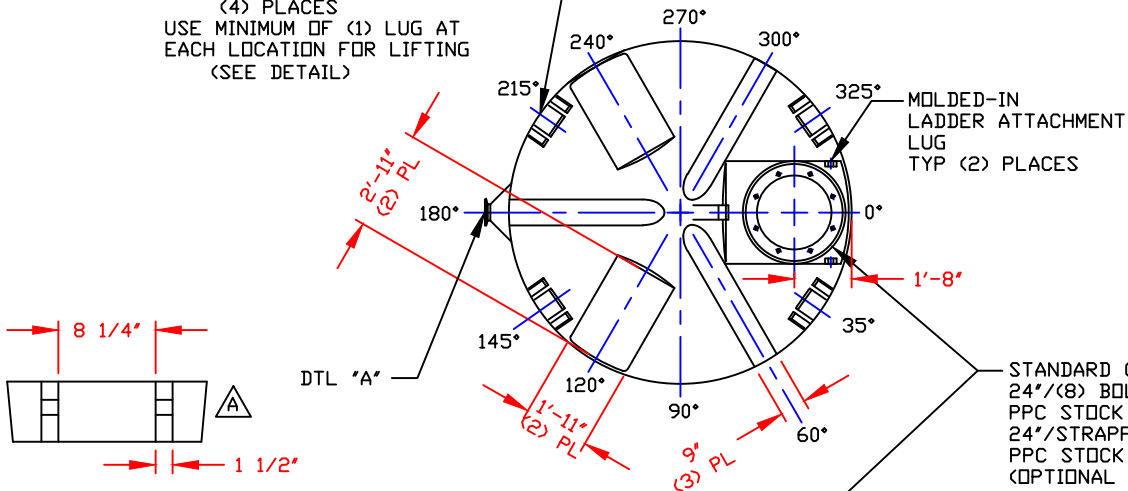
LIFTING LUG DETAIL (4) PLACES SCALE: 1"=1'-0"
